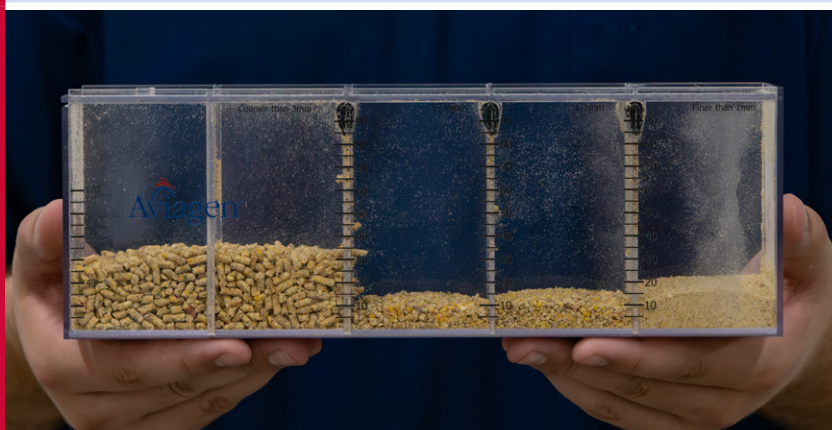
Рисунок 5.3 Пример сита-шейкера.
