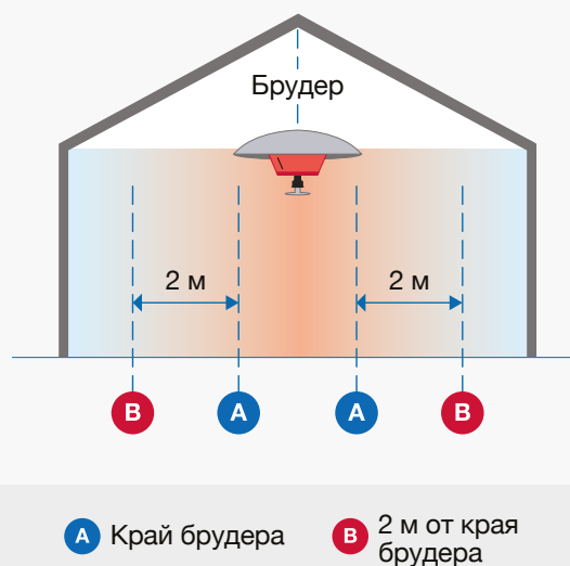
Рисунок 2.7 Градиция температуры при точечном брудерном содержании.
