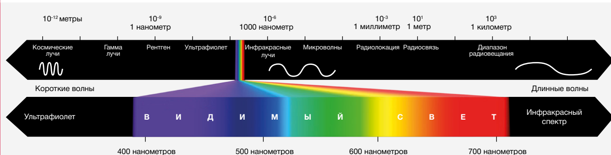
Рисунок 6.29 Световой спектр.
