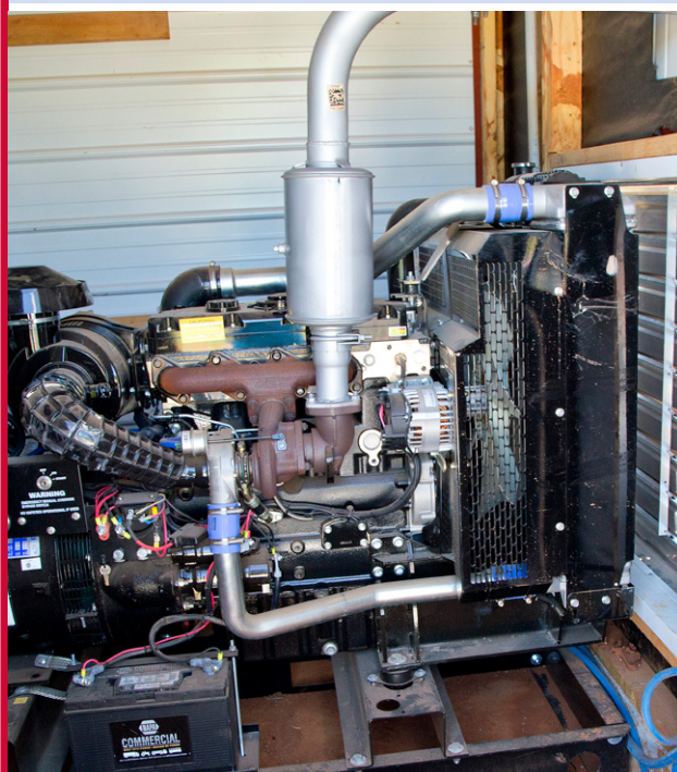
Рисунок 6.2 Пример запасного генератора.
