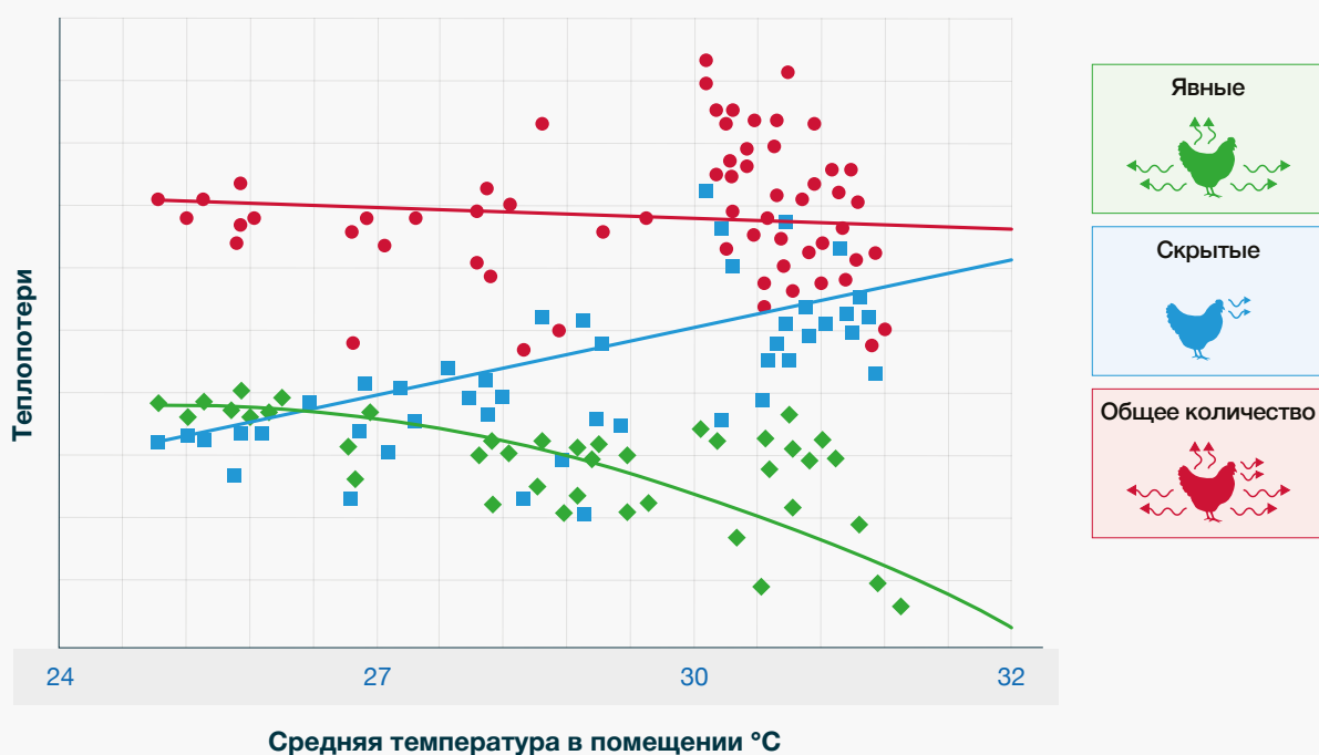
Рисунок 6.26 Явные и скрытые теплопотери.
